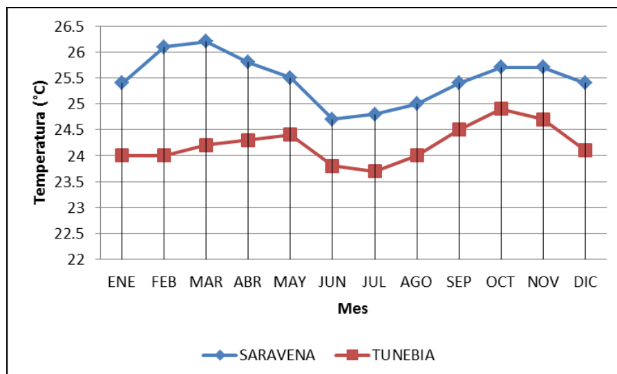
Figura 6 Variación temporal temperatura media multianual (°C) en Campo Arauca Fuente ECOPETROL S.A. 2011.
