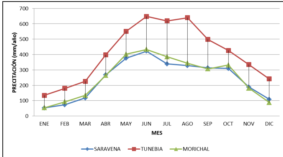
Figura 5 Variación temporal de la precipitación en Campo Arauca Fuente ECOPETROL S.A. 2011.
