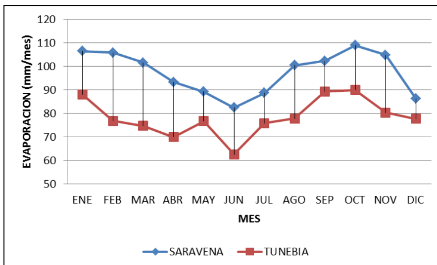
Figura 8 Variación temporal de la evaporación potencial (mm/año en Campo Arauca Fuente ECOPETROL S.A. 2011.
